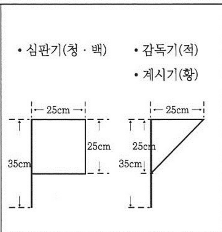
제5도(圖) 심판기 등의 규격
